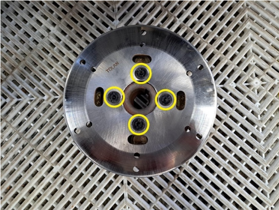
Irrota jarrulevyn kiinnityspultit. (kuusiokoloavain 5 mm).
